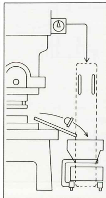
②カム入力・シャッター連動 Cam switch-shutter interlocking operation.
