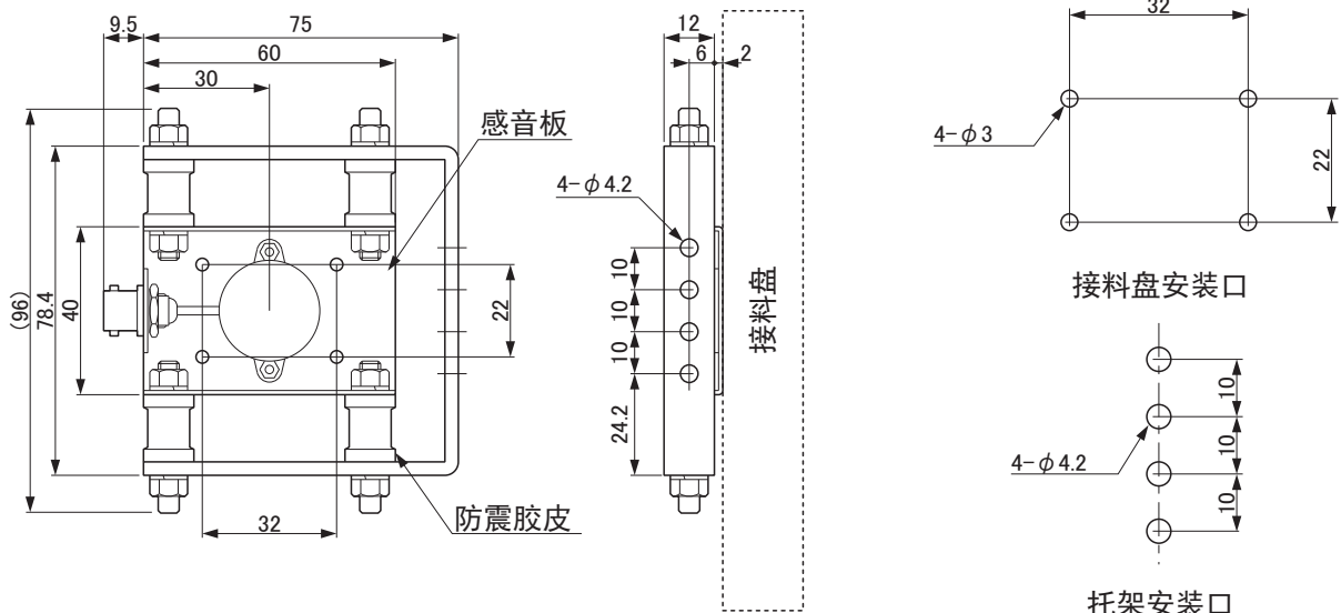
【AS-1102 传感头】
