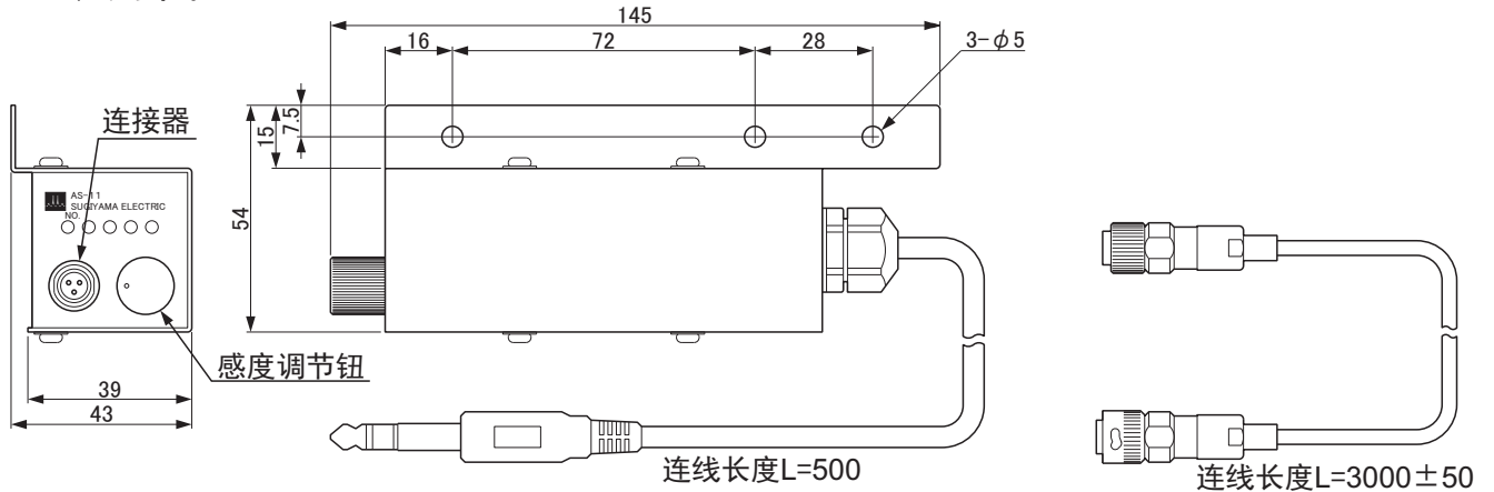
【AS-11 放大器】
