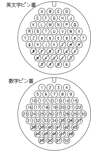
ピンコンタクト嵌合側からの図
