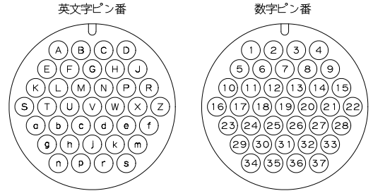
端子台信号割り当て
