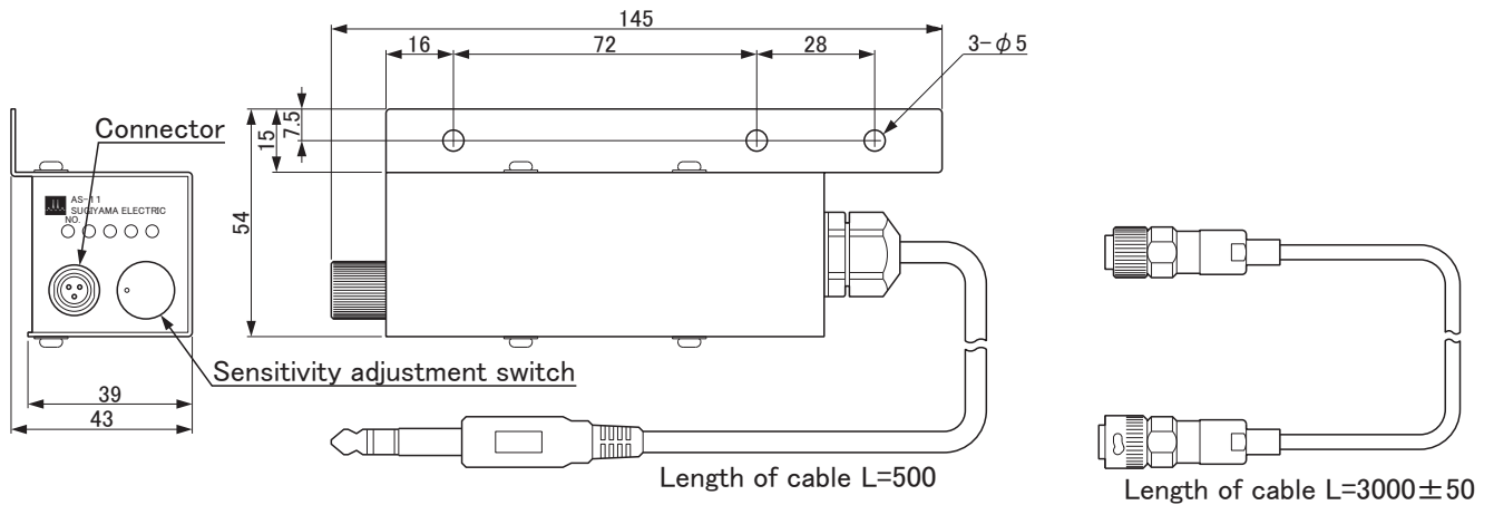
【AS-11 Amplifier】
